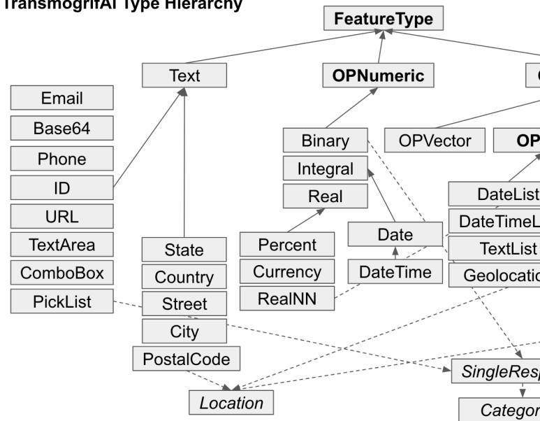
TransmogrifAI Type Hierarchy
